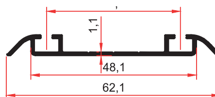
Οδηγός ντουλάπας Αλουμινίου Κάτω
