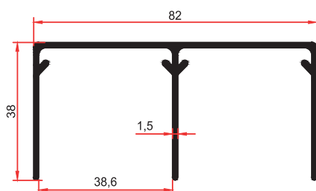
Οδηγός ντουλάπας Αλουμινίου Άνω
