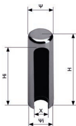
Καπάκι Βιδωτού Ρυθμιζόμενου
